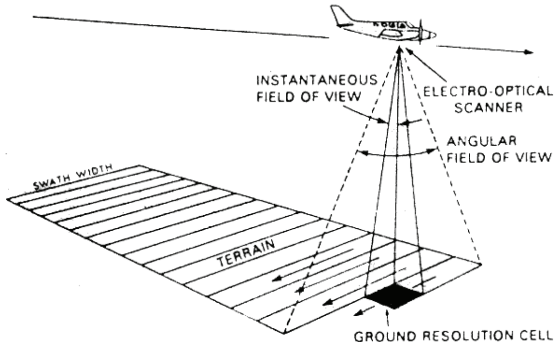
Fig. 1.25: AFOV
