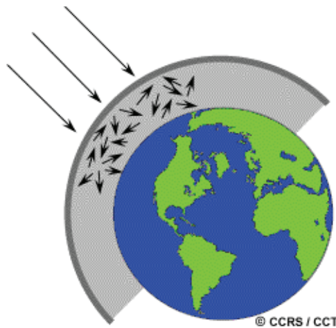
Fig. 1.10: Scattering
