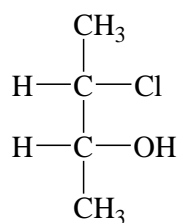
Erythro
