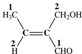
(E)-2-(hydroxymethyl)but-2-enal
