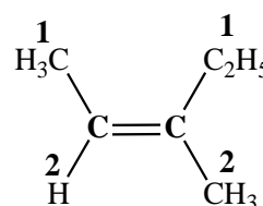
(Z)-3-methylpent-2-ene
