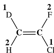
(E)-Deuterated 1-chloro-1-fluoroprop-1-ene
