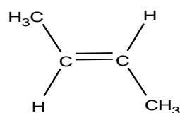
trans - But-2-ene
