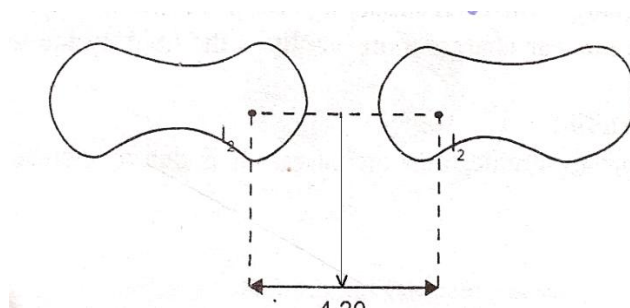
Fig. 3.3 van der Waals' radii
