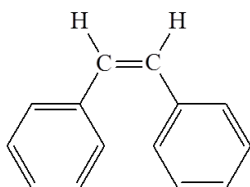
cis -stilbene
