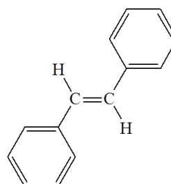
trans -stilbene
