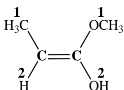
(Z)-1-methoxyprop-1-en-1-ol
