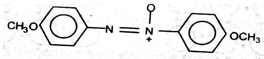
Fig 11.22 p-Ozoxyanisole
