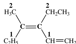
(Z)-3-ethyl-4-methylhexa-1,3-diene
