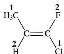
(E)-1-chloro-1-fluoroprop-1-ene
