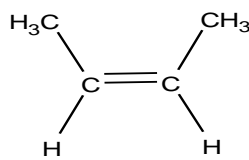
cis - But-2-ene
