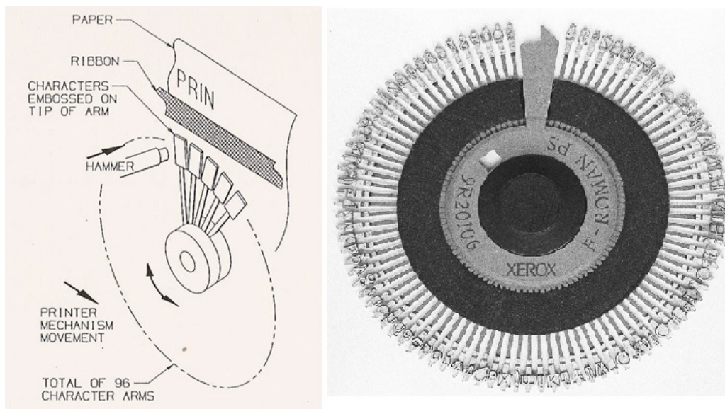
चित्र 3.11—डेजी व्हील प्रिंटर
